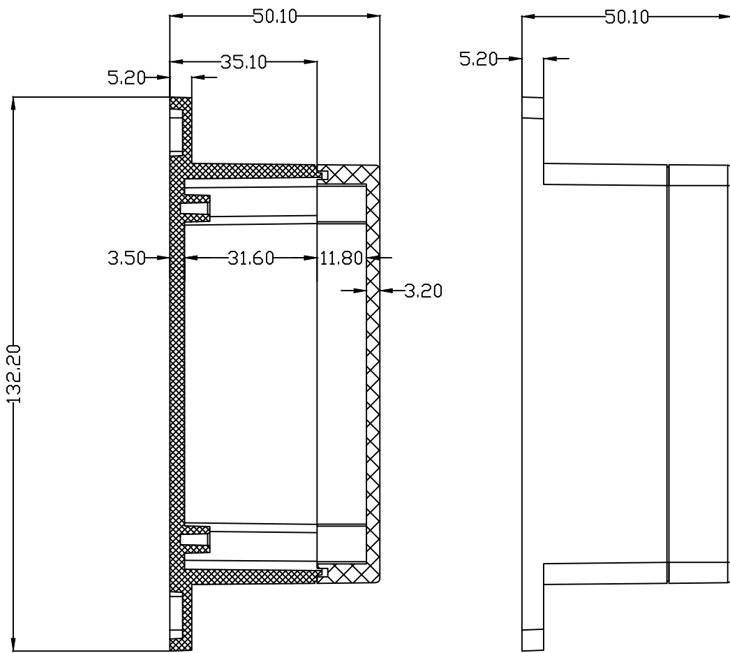
SECTION A-A
